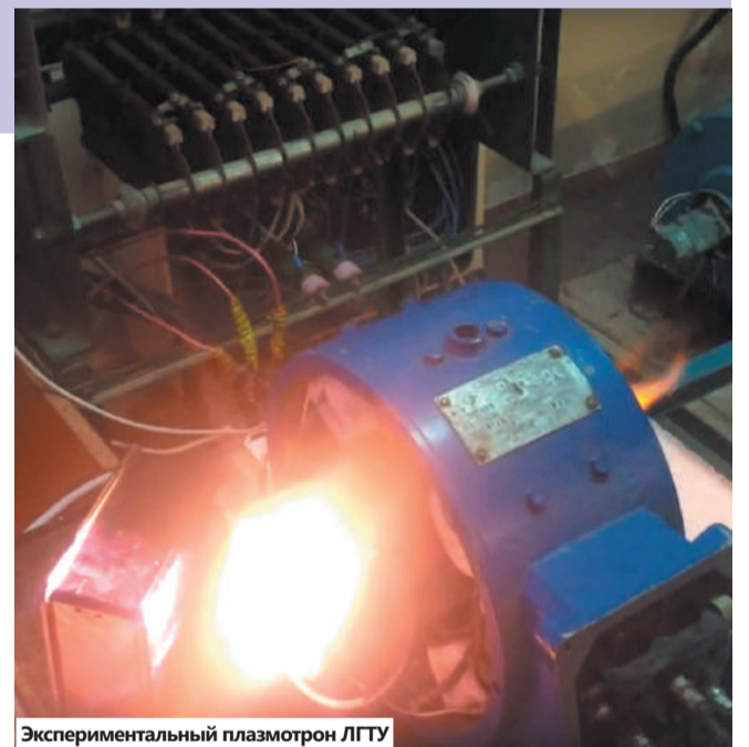
Экспериментальный плазмотрон ЛГТУ
